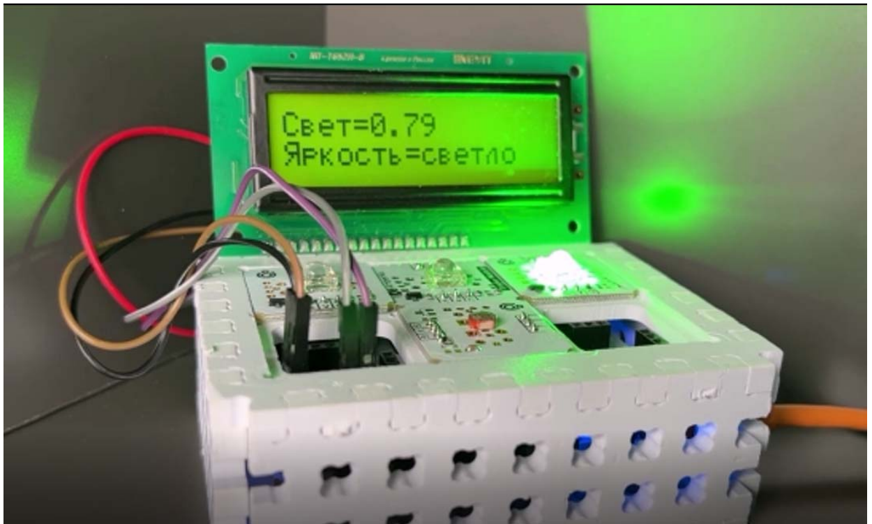
Датчик освещённости со световой индикацией
